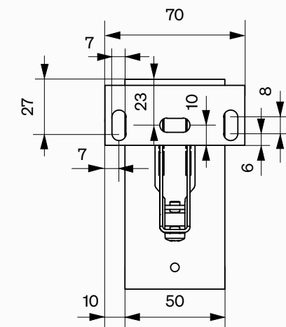
Halter Nr. 3S
