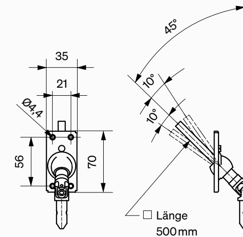
Durchführung Kurbel 45° (8 mm, 4-Kant Edelstahl) 35 × 70 mm
