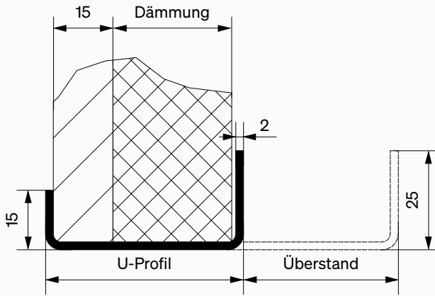
U-Profil mit Dämmung
