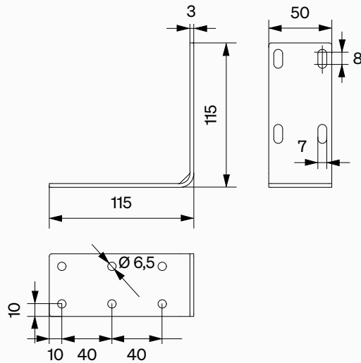
Ohne Wärmedämmung
