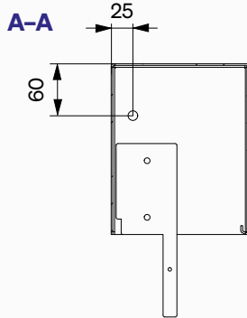
Seitenteil links
