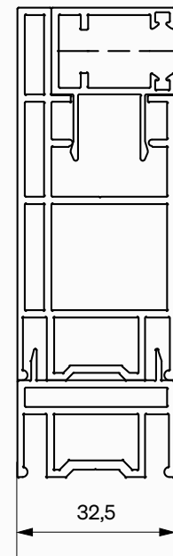
Versatz
