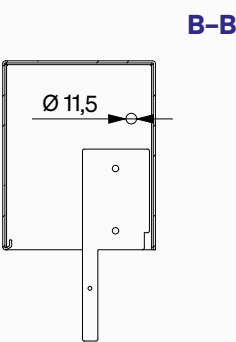
Seitenteil rechts
