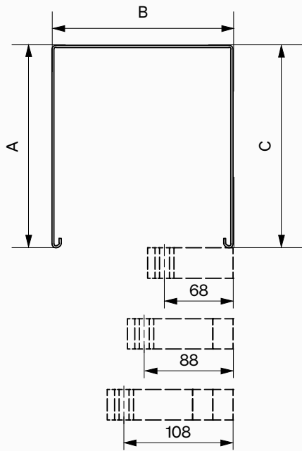
Blenden ohne Biegung D (F11, F21, F30, F33)
