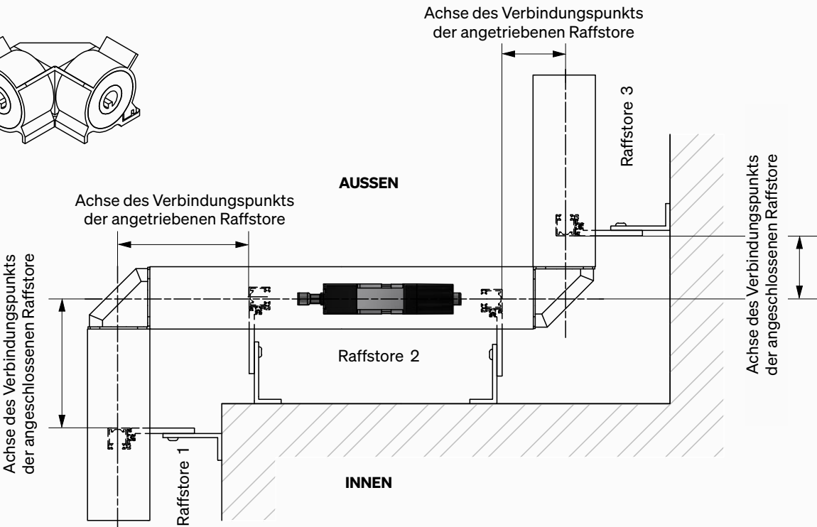
Eckkupplung 90°
