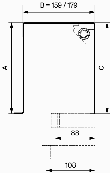
Blende Typ F11
