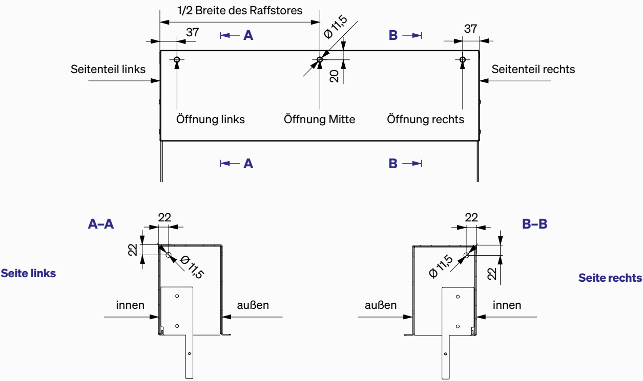
Öffnungen – Rückseite der Blende / Ansicht von innen
