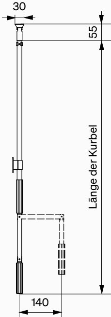
Abnehmbare Kurbel
