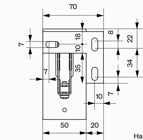
Halter Nr. 3P
