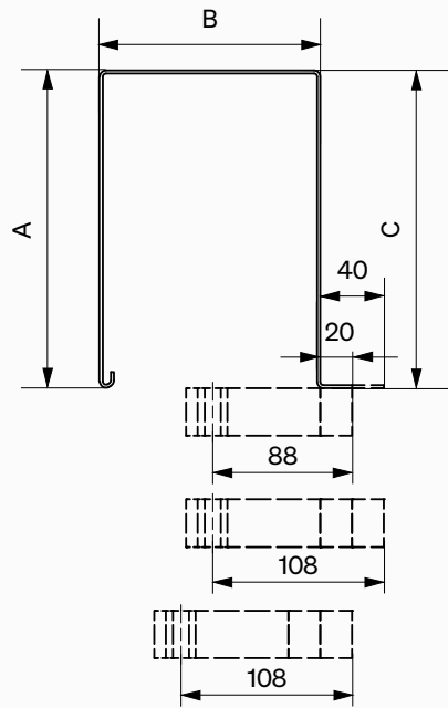
Blenden mit Biegung D (F31, F32)
