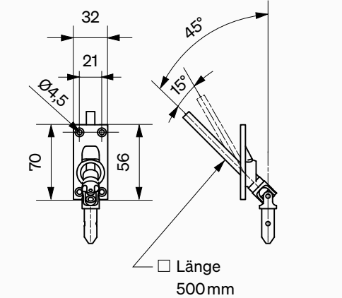
Eckdurchführung Kurbel (4 mm, 4-Kant)
