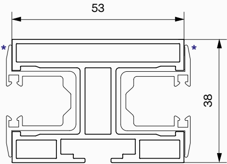
Typ STL DV-Doppeltyp
