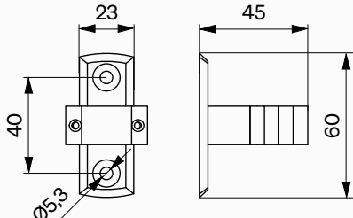
Rohrlager für Kurbel
