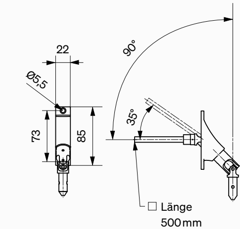
Durchführung Kurbel 45° (8 mm, 4-Kant Kunststoff) 25 × 90 mm
