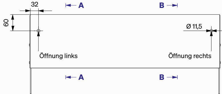
Öffnungen – Rückseite der Blende / Ansicht von innen
