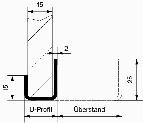
U-Profil ohne Dämmung
