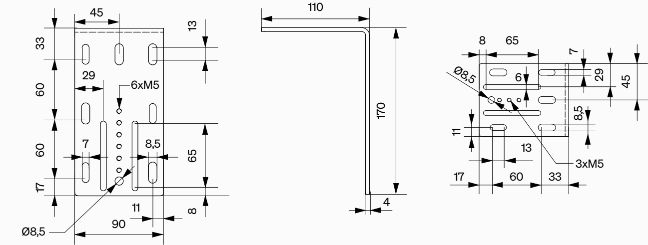
Halter Nr. 52
