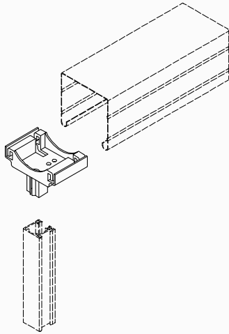
Kunststoff-Halter
