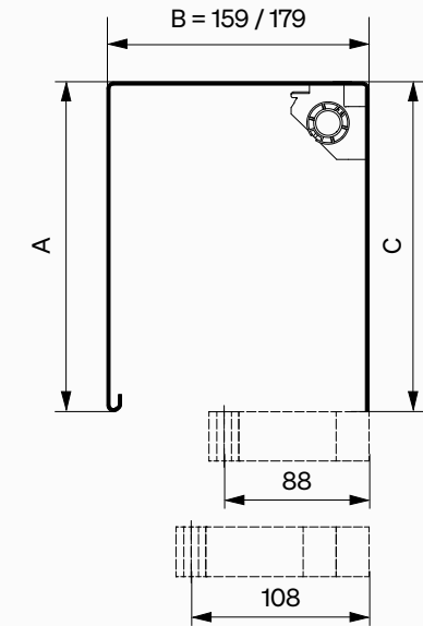
Blende Typ F21
