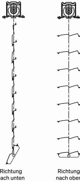
Raffstore S90, Z90, Z70 (einseitig)
