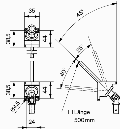
Eckdurchführung Kurbel (4 mm, 4-Kant)
