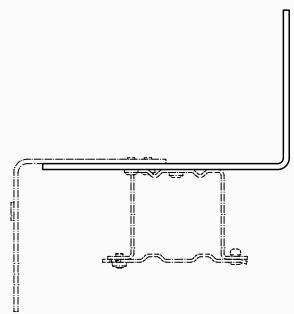
Halter Nr. 5
