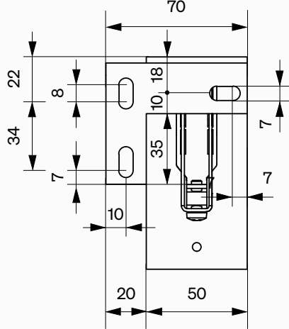
Halter Nr. 3L
