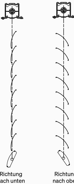
Raffstore C80, C65, F80 (beidseitig)
