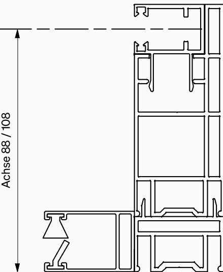
Ohne Versatz
