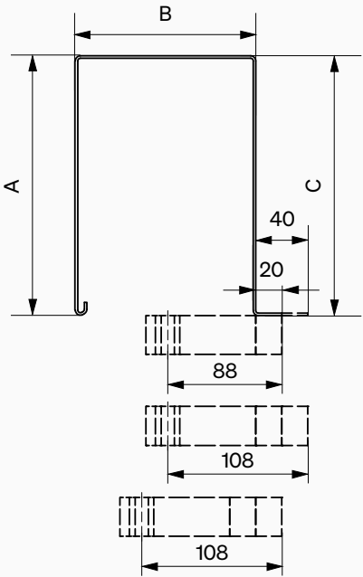
Lambrequins avec pliage en D (F31, F32)
