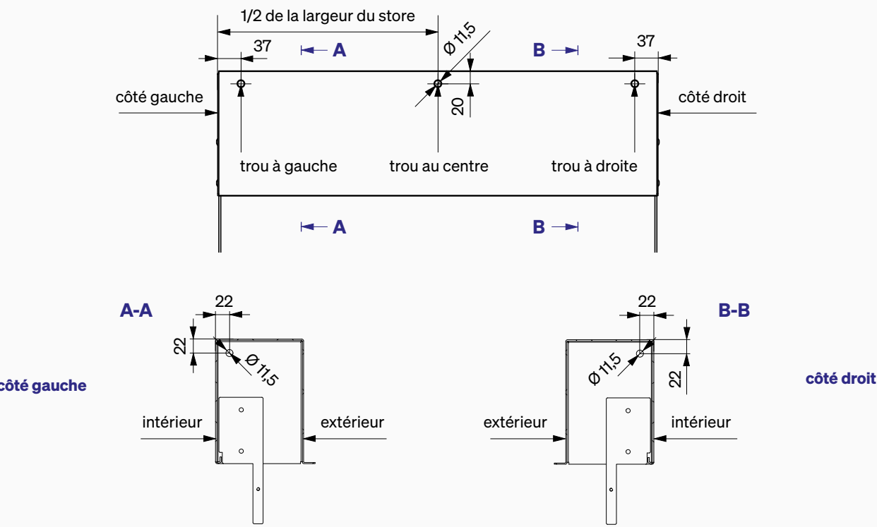
Trous - côté arrière du lambrequin / vue de l'intérieur
