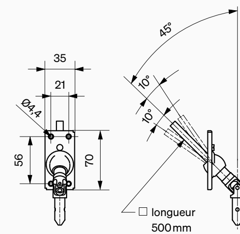
Passage de la manivelle 45° (8 mm, 4 bords inox) 35×70 mm
