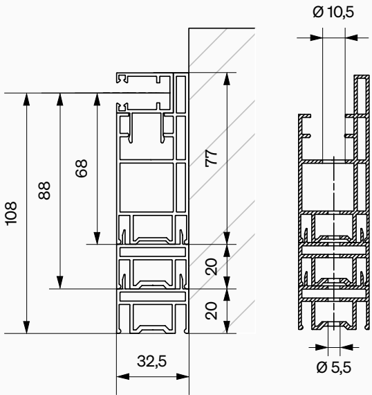
STF1 + trous de montage
