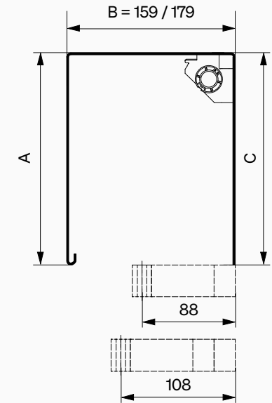
Lambrequin de type F21
