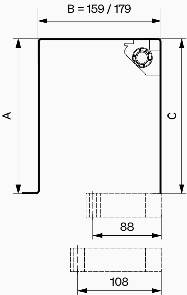
Lambrequin de type F11
