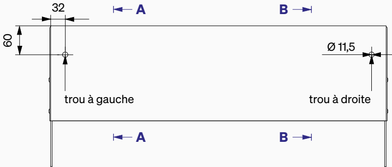
Trous - côté arrière du lambrequin / vue de l'intérieur
