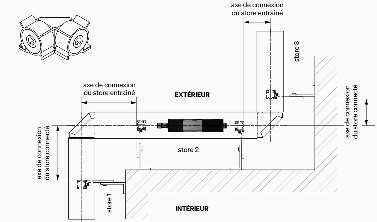
Accouplement d'angle 90°
