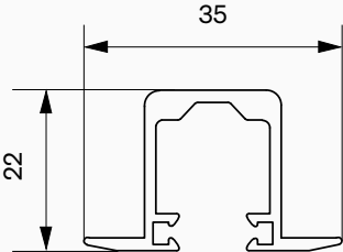
Type Z — pour STF2, STL, STL DV, coulisseau, ISO-PANEL
