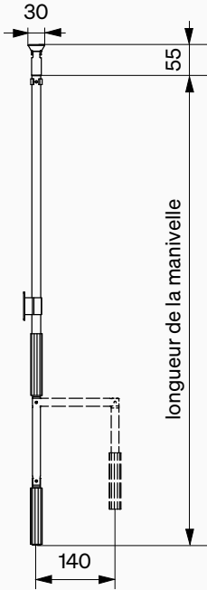
Manivelle amovible
