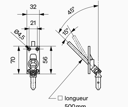
Passage de la manivelle d'angle (4 mm, 4 bords)
