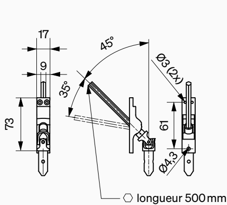
Passage de la manivelle à 45° (6mm, 6 bords)
