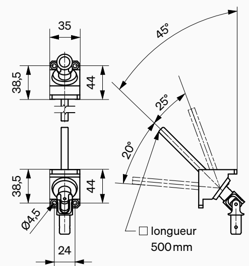
Passage de la manivelle d'angle (4 mm, 4 bords)
